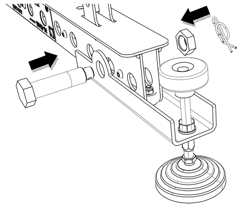
1 b Attacher un M-JACK dans le deuxième trou d'une M-BAR.
