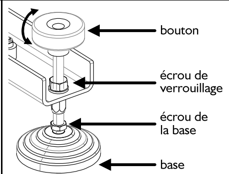
4 Ajuster la hauteur du M-JACK
