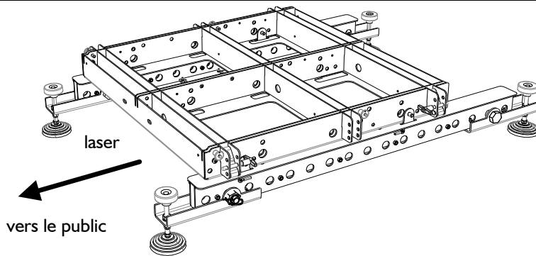
3 La plateforme de pose en extension arrière
