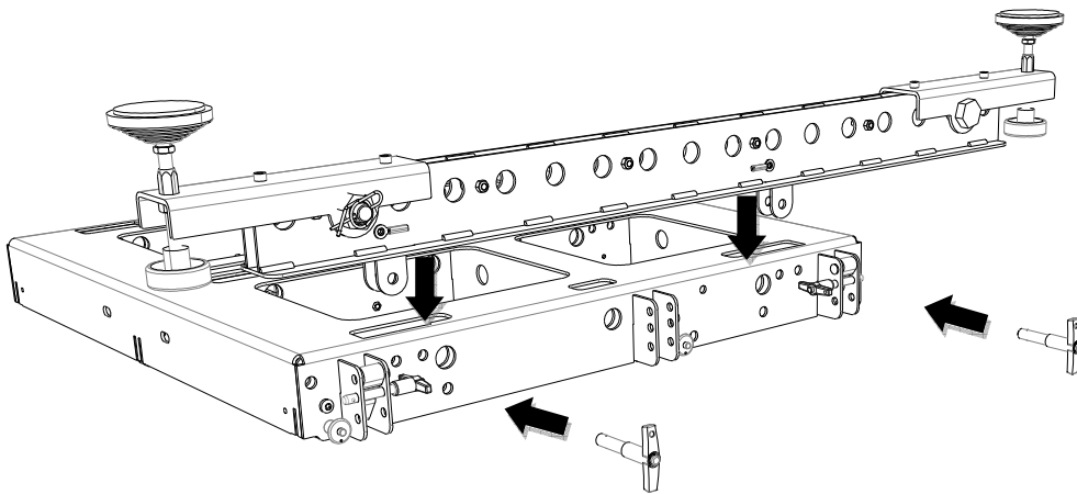
2 Attacher un assemblage M-BAR/M-JACK à un M-BUMP en extension arrière (position A ou B).
