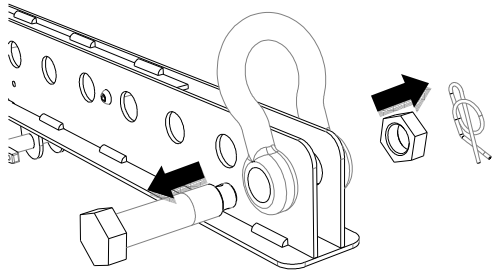
1 a Retirer une manille d'une M-BAR.
