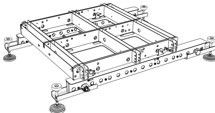
FIN La plateforme M-BUMP prête pour les enceintes.
